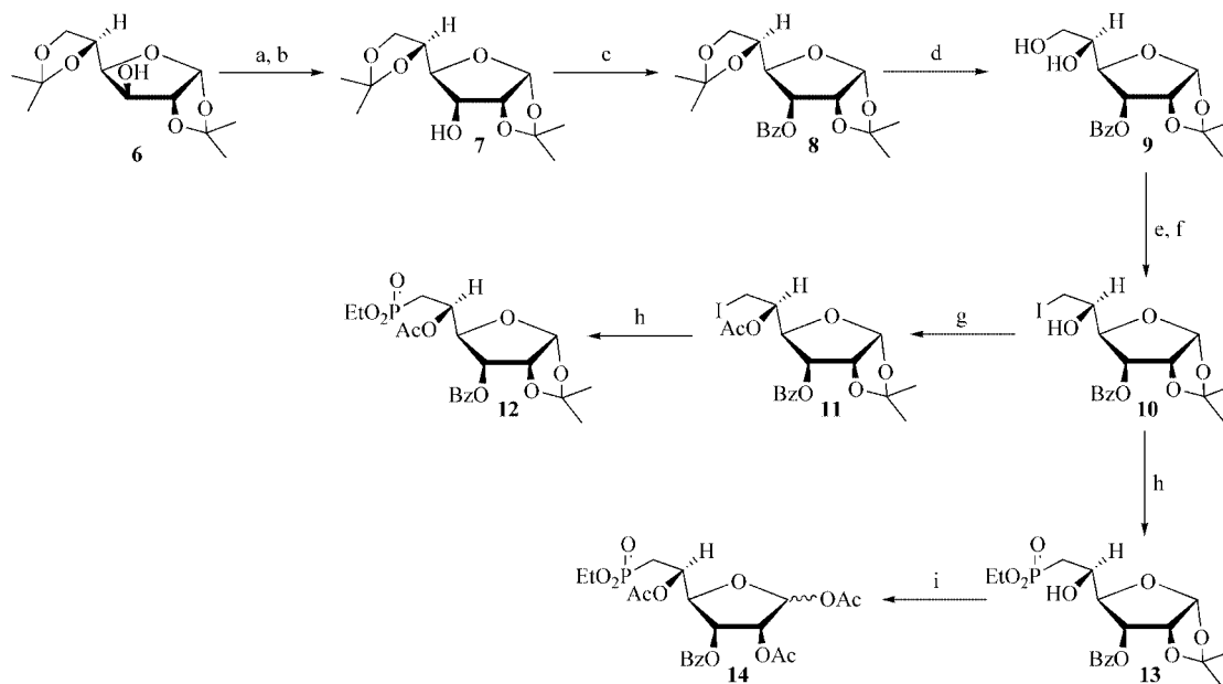
Scheme 2. Preparation of key “sugar-phosphonate” intermediate 14. a) CrO 3 , Ac 2 O, pyr., CH 2 Cl 2 ; b) NaBH 4 , EtOH abs ; c) BzCl, pyr.; d) AcOH aq 90%, 60 °C; e) TsCl, DMAP, pyr.; f) NaI, acetone, reflux; g) Ac 2 O, pyr.; h) P(OEt) 3 , 110 °C or MW irradiation; i) Ac 2 O, AcOH, conc. H 2 SO 4 .
